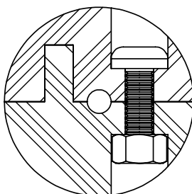
KESIT A-A
